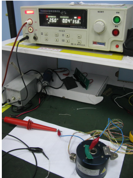
← 对控制地测试
