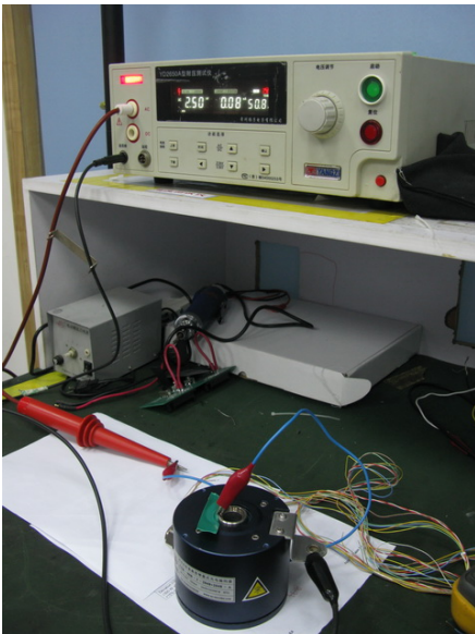
← 对机壳地测试
